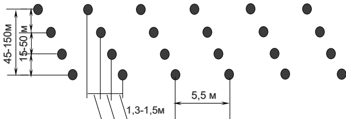
Мал. 2. Схема 4-рядного ПТМП з протигусеничних мін.
