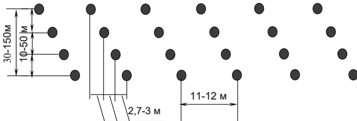
Мал. 4. Схема 4-рядного ПТМП з протицивільних мін.
