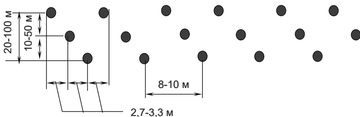
Мал. 3. Схема 3-рядного ПТМП з протицивільних мін.
