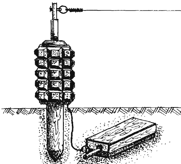
Рис. 6.2. Встановлення ПОМЗ-2 по нестандартній схемі (невилучене становище)
